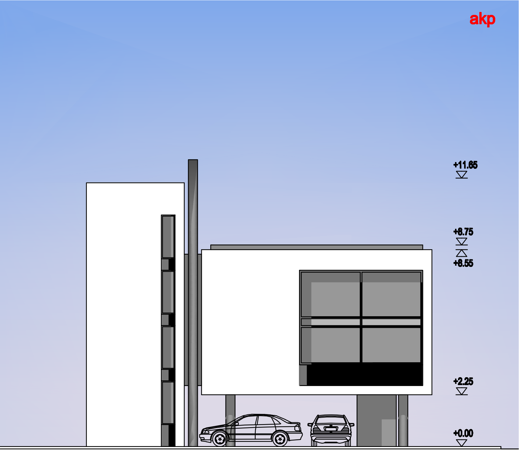
POHĽAD JUHOVÝCHODNÝ - KOPČIANSKA ULICA
